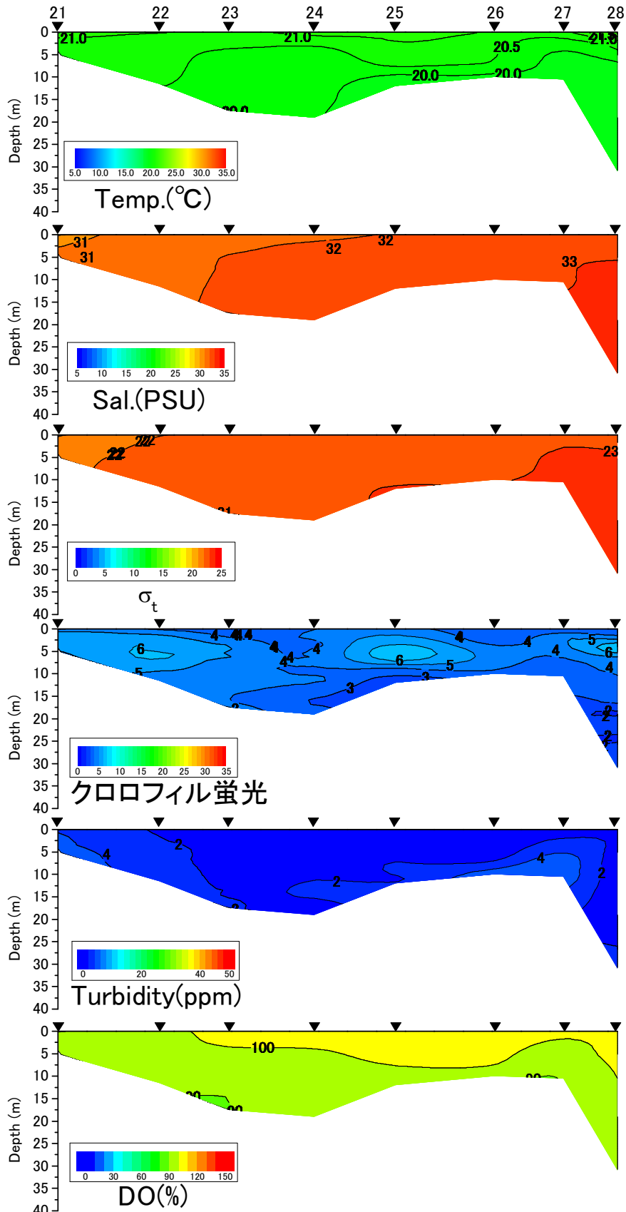
有明海東ラインの水温(°C)、塩分、密度( \sigma_t )、クロロフィル蛍光強度、濁度、溶存酸素飽和度(DO%)の鉛直面図(国土交通省の調査による) (2014年5月29日)
